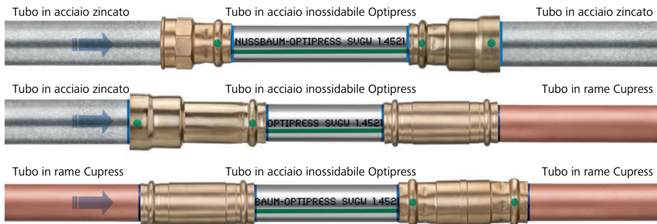
Fig. 4: Installazioni miste consentite con Optipress-Aquaplus
