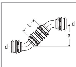
Curva 45° Optiflex-Flowpress 84241
