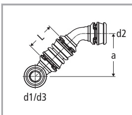
Pezzo a T Optiflex-Flowpress con curva 45° Optiflex-Flowpress 84242/84241
