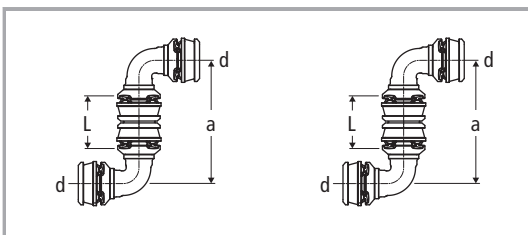
Curva 90° Optiflex-Flowpress 84240
