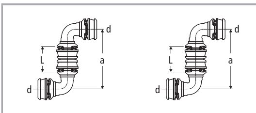
Curva 90° Optiflex-Flowpress 84240
