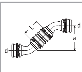
Curva 45° Optiflex-Flowpress 84241
