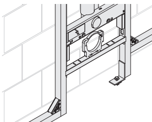
Fig. 35: Fixation du module avec une équerre de fixation, le profilé de sol étant interrompu
