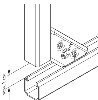
Fig. 24: Tolérances pour la coupe sur mesure des profilés Optivis-Tec
