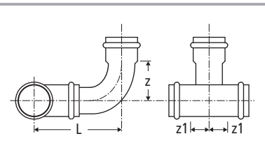
Combinaison Optipress-Therm 55010 / 55001
