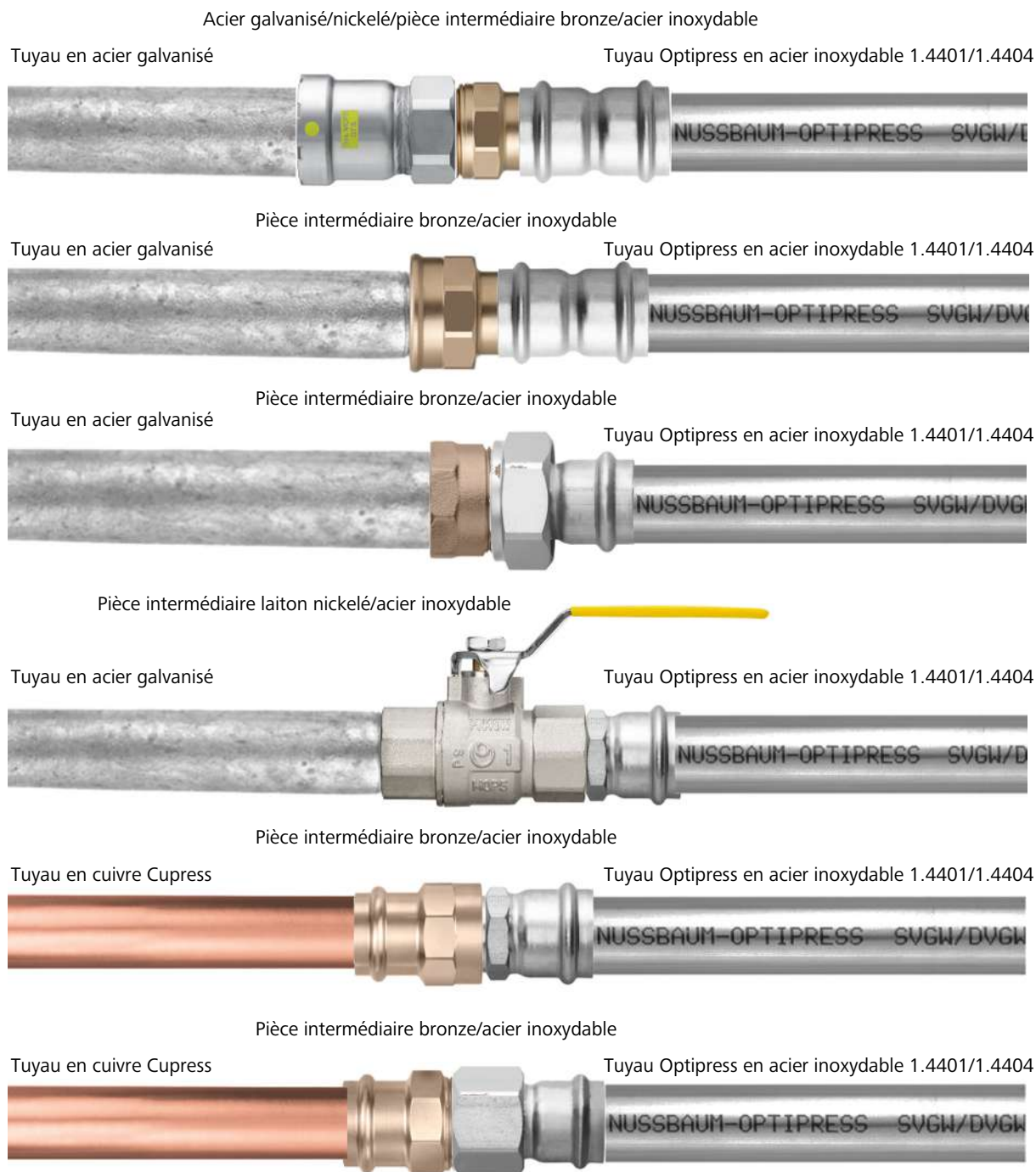
Fig. 3: Installations mixtes admissibles avec Optipress-Gaz
