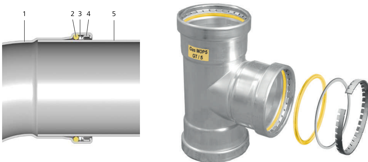
Fig. 2: Assemblage par sertissage Optipress-Gaz-XL Ø 64, 76.1, 88.9 et 108 mm
