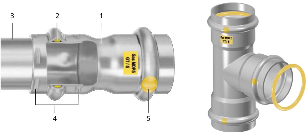
Fig. 1: Assemblage par sertissage Optipress-Gaz jusqu'à Ø 15 à 54 mm
