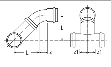
Combinaison Optipress-Aquaplus 80010 / 80004
