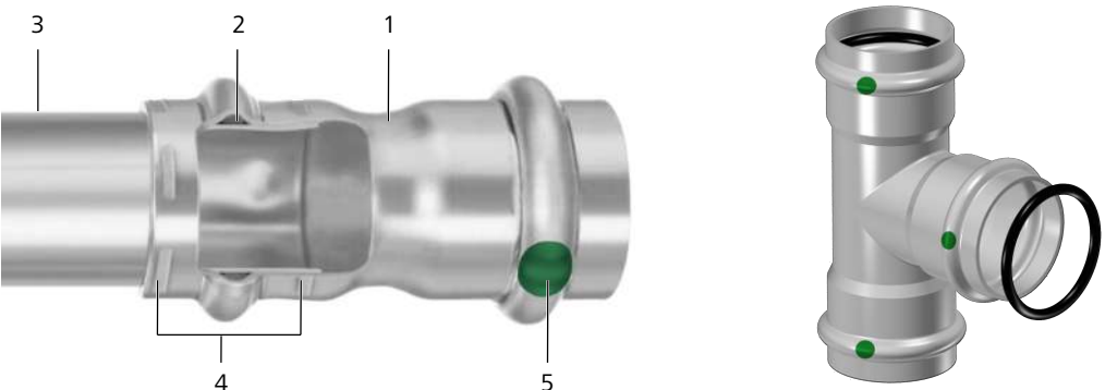
Fig. 1: Assemblage par sertissage Optipress-Aquaplast jusqu'à Ø 15 à 54 mm
