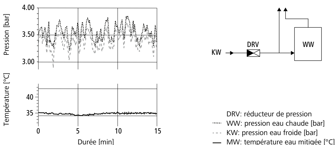
Fig. 1: Variations mineures de la température aux points de soutirage (eau mitigée) du fait d'un montage en amont du réducteur de pression
