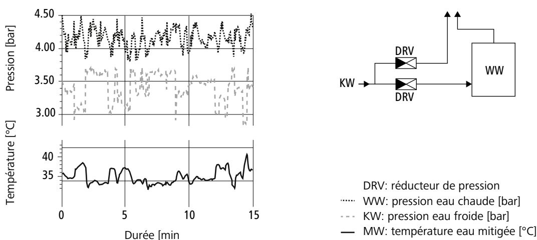
Fig. 2: Variations importantes de la température aux points de soutirage (eau mitigée) du fait d'un montage en aval du réducteur de pression
