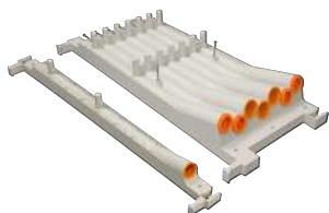
Optiflex-Liste d'évidement sur coffrage 87054
