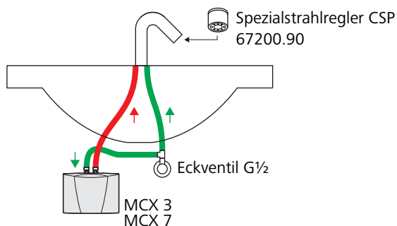
Abb. 1: Montagebeispiel Untertischmontage
