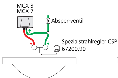
Abb. 2: Montagebeispiel Übertischmontage
