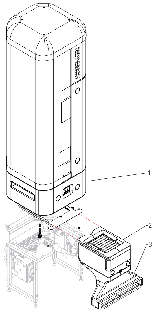
Abb. 1: 68000.21 Gerät mit Armatureneinheit 68080 erhältlich, für Schrankeinbau SMS / SN EN 1116:2018
