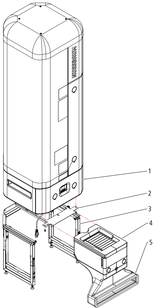
Abb. 2: Gerät 68010, für Schrankeinbau SMS / SN EN 1116:2018
