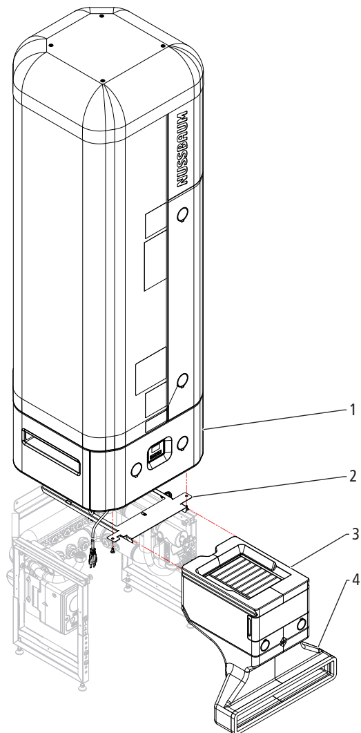
Abb. 1: Gerät 68000.21, für Schrankeinbau SMS / SN EN 1116:2018, erhältlich mit Armatureinheit 68080
