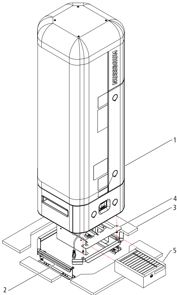
Abb. 1: Austauschgerät 68020.22, für Schrankeinbau, mit Aufsatz für Fremdgestell
