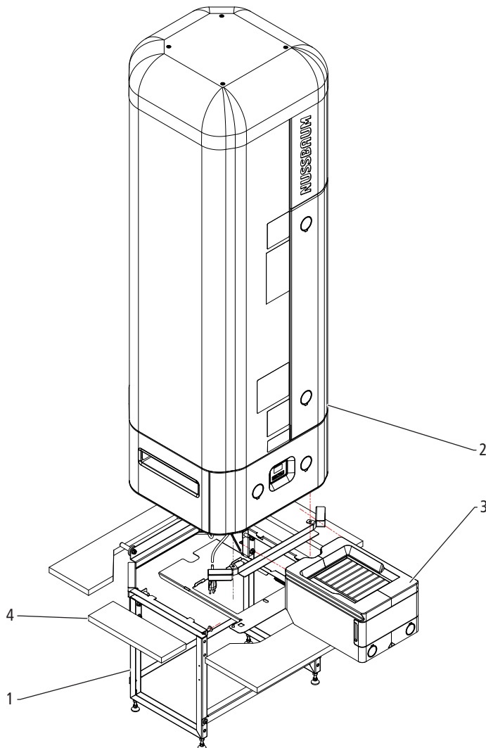
Abb. 1: 68020.21 Austauschgerät für Schrankeinbau, mit Nussbaum Unterbau
