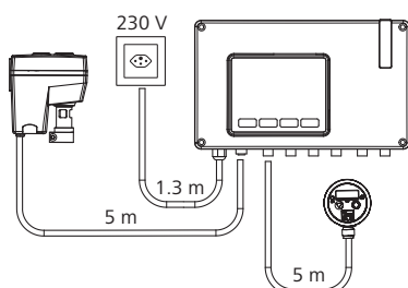
Abb. 9: Kabellängen
