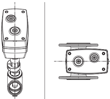
Abb. 7: Bevorzugte Montagepositionen
