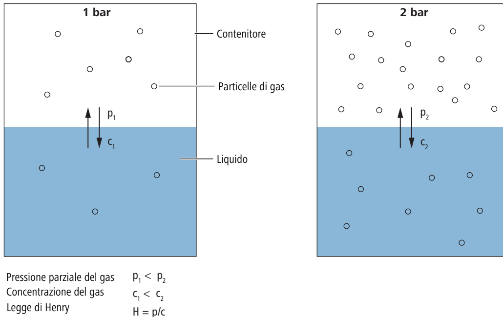
Fig. 3: Legge di Henry
