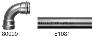
Fig. 4: Coude Optipress-Aquaplus 90° et tuyau en acier inoxydable Optipress 1.4520
