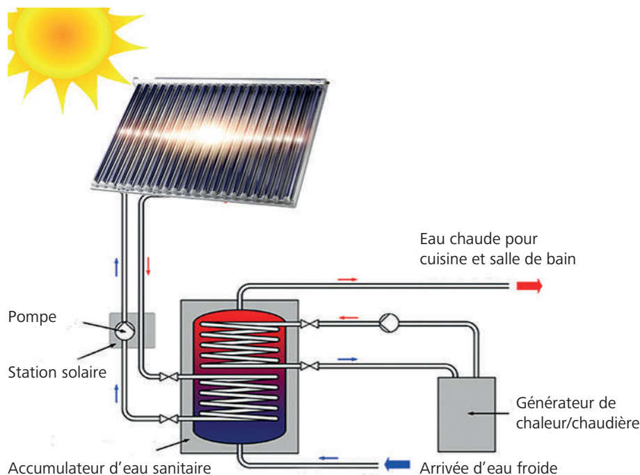
Fig. 1: Schéma d'une installation solaire thermique
