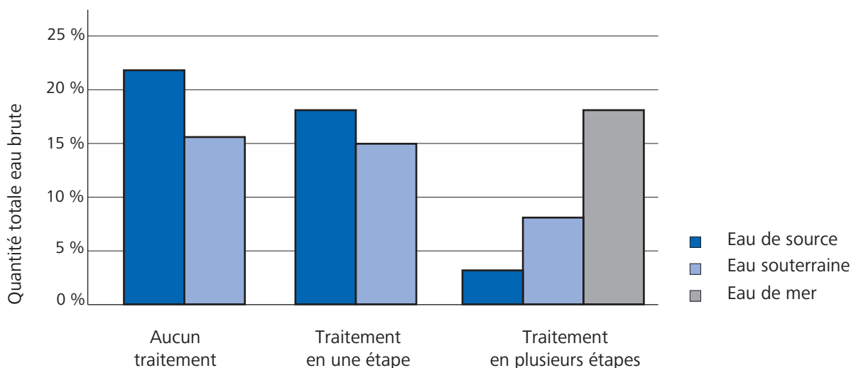
Fig. 4: Comparaison de l'énergie nécessaire au traitement des eaux brutes
