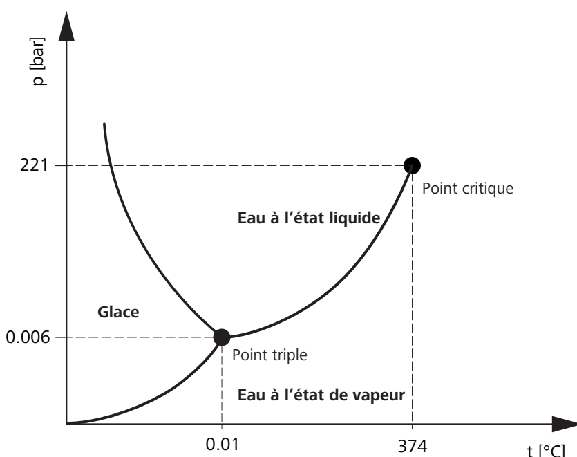
Fig. 1: Diagramme de phase de l'eau
