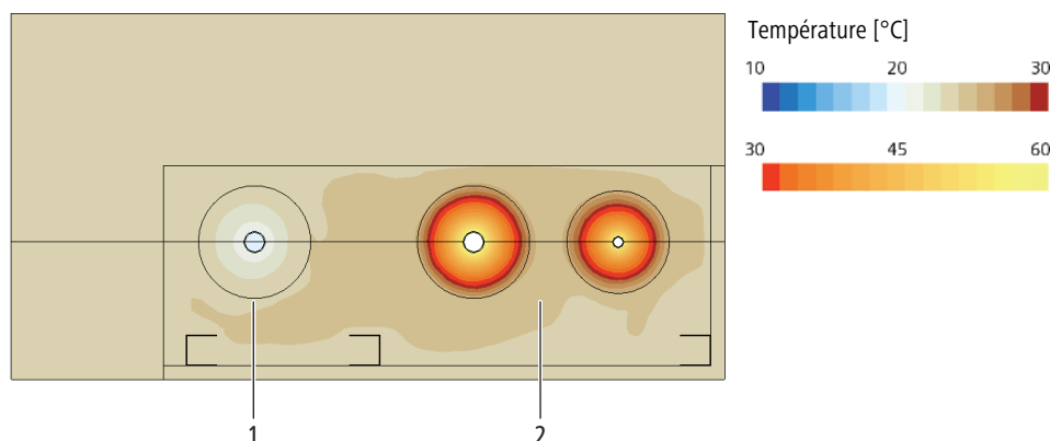
Fig. 33: Visualisation de la distribution de température dans une simulation de gaine montante sans flochage de la gaine, distribution de la chaleur après 12 heures de stagnation, température PWC 21 °C, distance axiale entre colonne montante PWC et PWH 15 cm, température ambiante 23 °C
