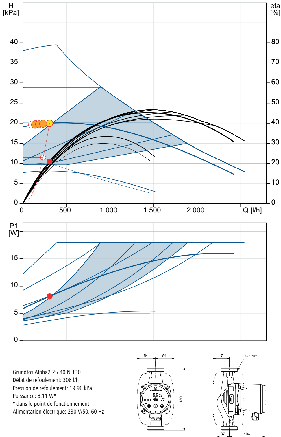
Fig. 42: Choix de la pompe de circulation à l'aide de l'outil de calcul du fabricant (figures: Grundfos)
