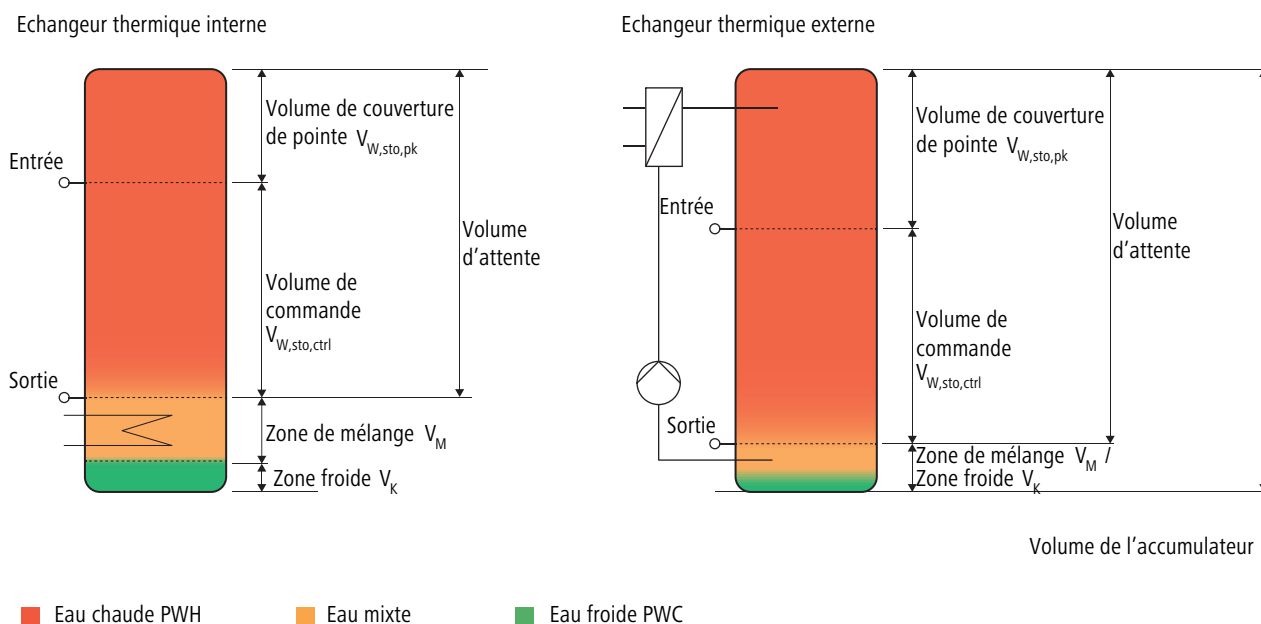
Fig. 15: Stratification dans le chauffe-eau à accumulation avec échangeur de chaleur interne et externe
