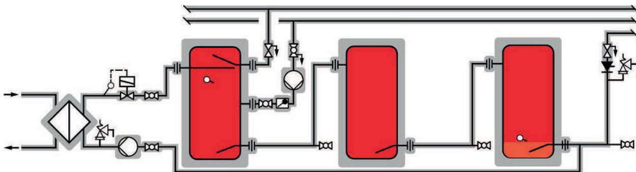
Fig. 14: Raccordement en série de trois chauffe-eau à accumulation
