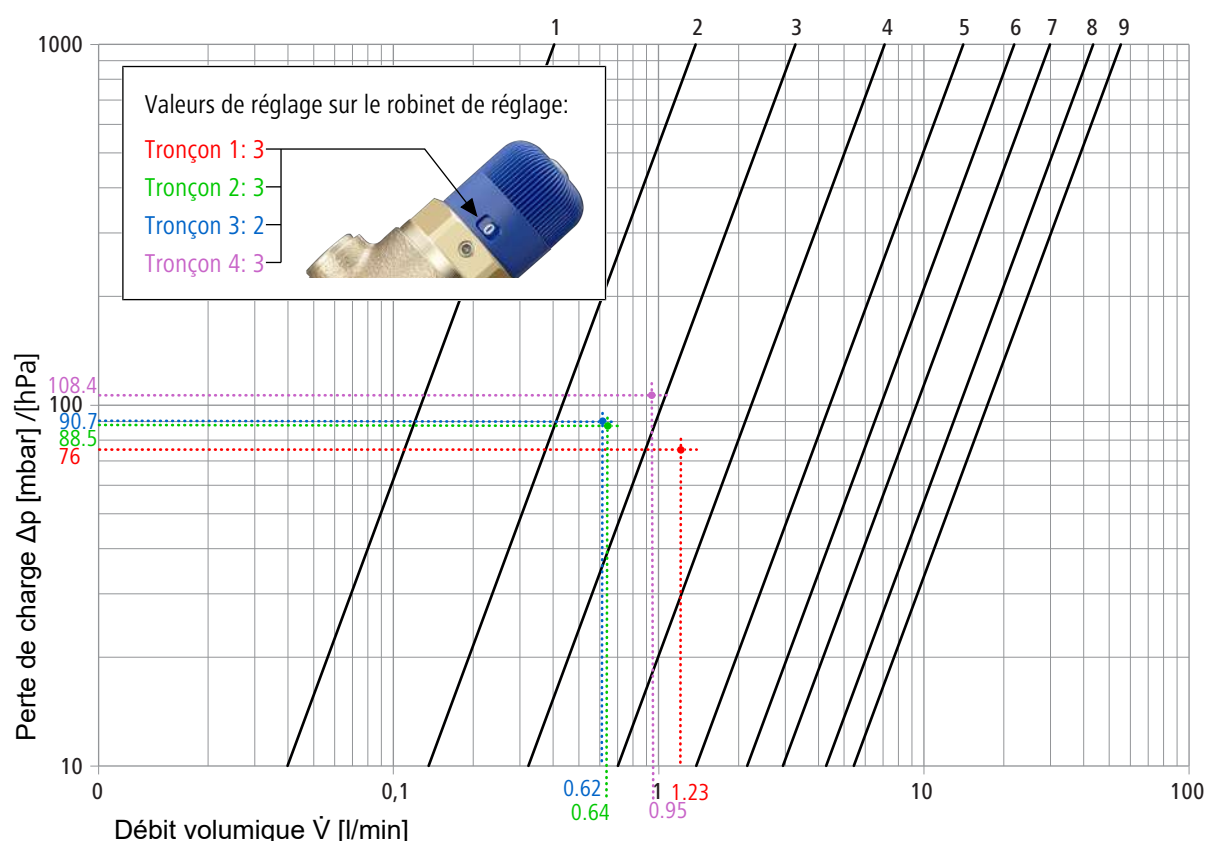
Fig. 43: Exemples de lecture pour le diagramme du robinet de réglage 24025
