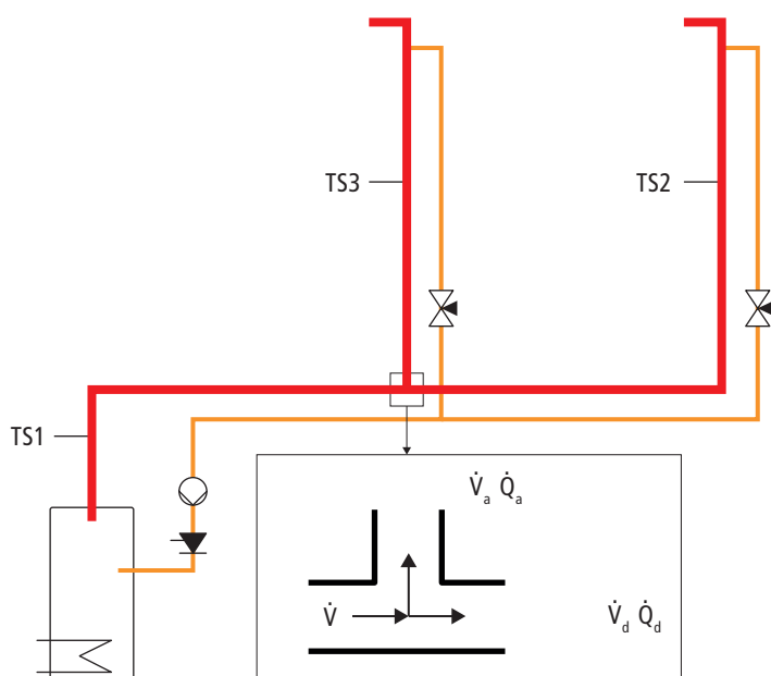
Fig. 36: Calcul des débits volumiques (selon le cours sur l'eau de suisselec)
