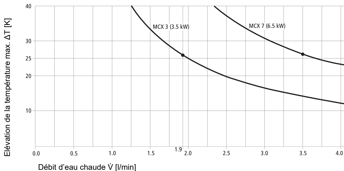
Fig. 19: Diagramme de performance d'un chauffe-eau instantané (exemple)
