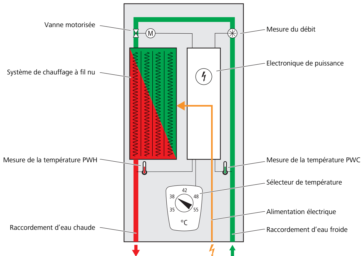
Fig. 18: Principe de fonctionnement d'un chauffe-eau instantané à régulation électronique
