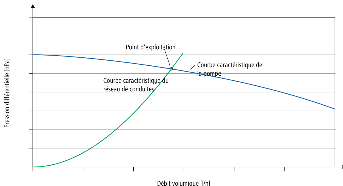
Fig. 37: Courbe caractéristique de la pompe, courbe caractéristique du réseau de conduites et point d'exploitation
