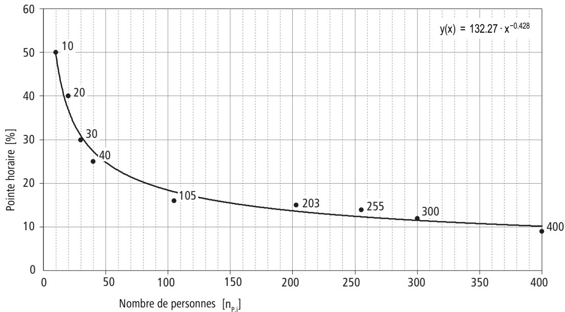
Fig. 35: Pointe horaire pour immeubles résidentiels > 10 personnes (selon calculs sanitaires – brefs et précis)
