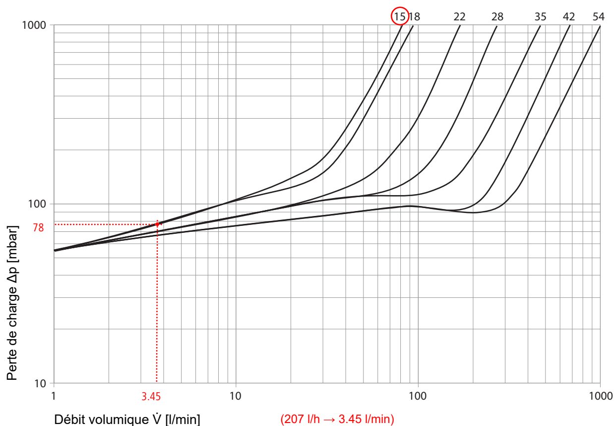
Fig. 40: Exemple de lecture pour le diagramme de performance du clapet anti-retour Optipress-Aquaplus 80189/81163
