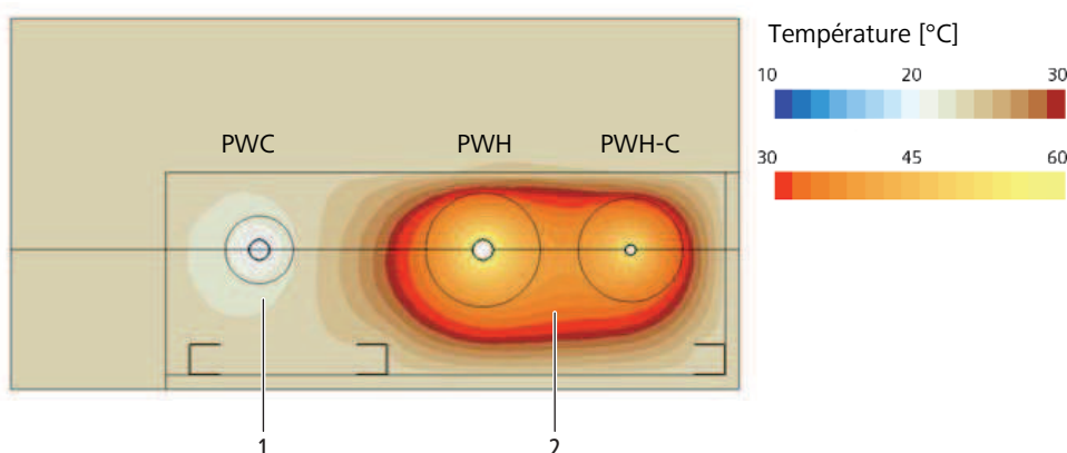
Fig. 34: Visualisation de la distribution de température dans une simulation de gaine floquée après 12 heures de stagnation, température PWC 23 °C, distance axiale entre colonne montante PWC et PWH 15 cm
