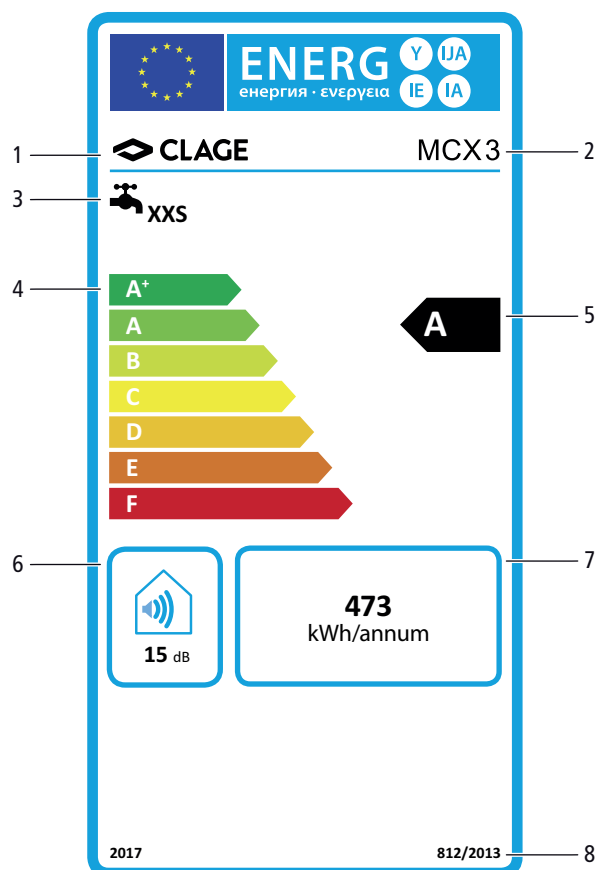
Fig. 46: Indication de la consommation d'énergie du chauffe-eau instantané pour lavabo MCX 3
