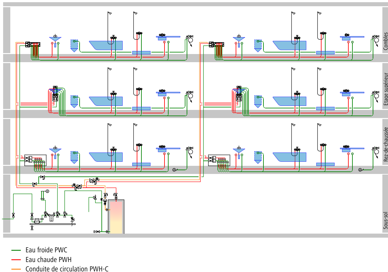
Fig. 24: Approvisionnement centralisé en eau chaude avec circuit de circulation d'eau chaude
