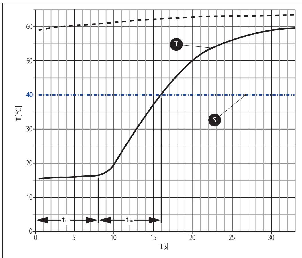
Fig. 44: Evolution de la température sur un point de soutirage d'eau chaude
