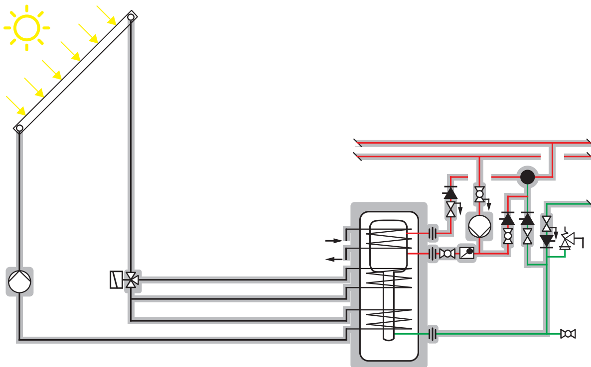
Fig. 13: Chauffe-eau à accumulation avec accumulateur tampon (accumulateur mixte)
