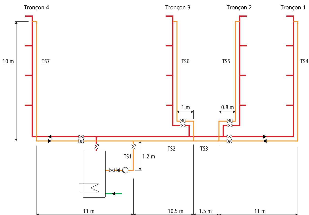
Fig. 38: Exemple de dimensionnement de la circulation d'eau chaude (selon le cours sur l'eau de swissetec)
