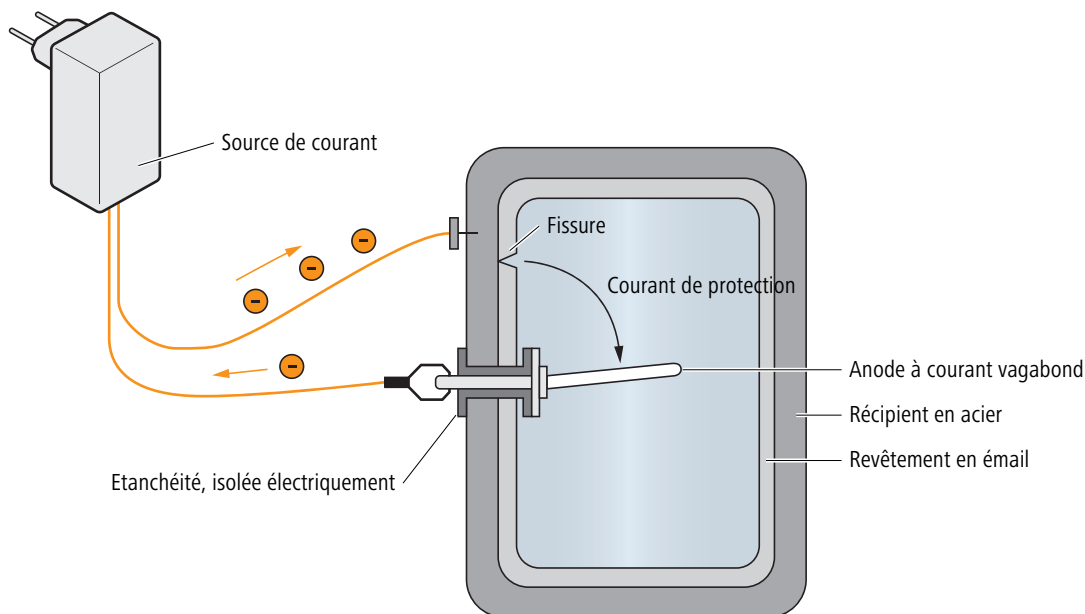
Fig. 17: Anode à courant vagabond (schéma: Blickle, Technique d'installation)
