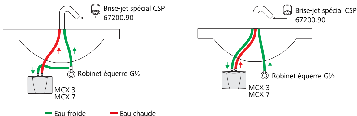
Fig. 21: Approvisionnement individuel doté d'un chauffe-eau instantané pour lavabos MCX 3 / MCX 7
