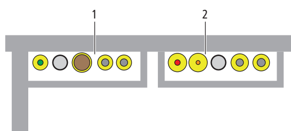
Fig. 30: Gaines d'installation séparées
