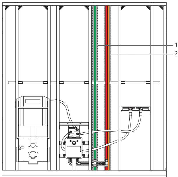
Fig. 32: Colonne montante d'eau froide à isolation renforcée dans un système de cadres de montage
