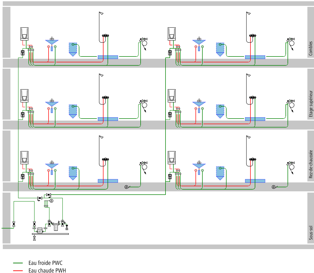
Fig. 22: Alimentation groupée avec chauffe-eau instantanés
