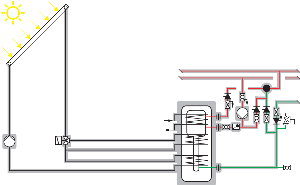
Fig. 13: Chauffe-eau à accumulation avec accumulateur tampon (accumulateur mixte)
