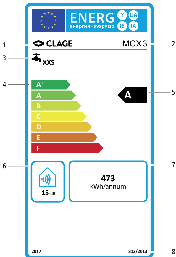
Fig. 44: Indication de la consommation d'énergie du chauffe-eau instantané pour lavabo MCX 3
