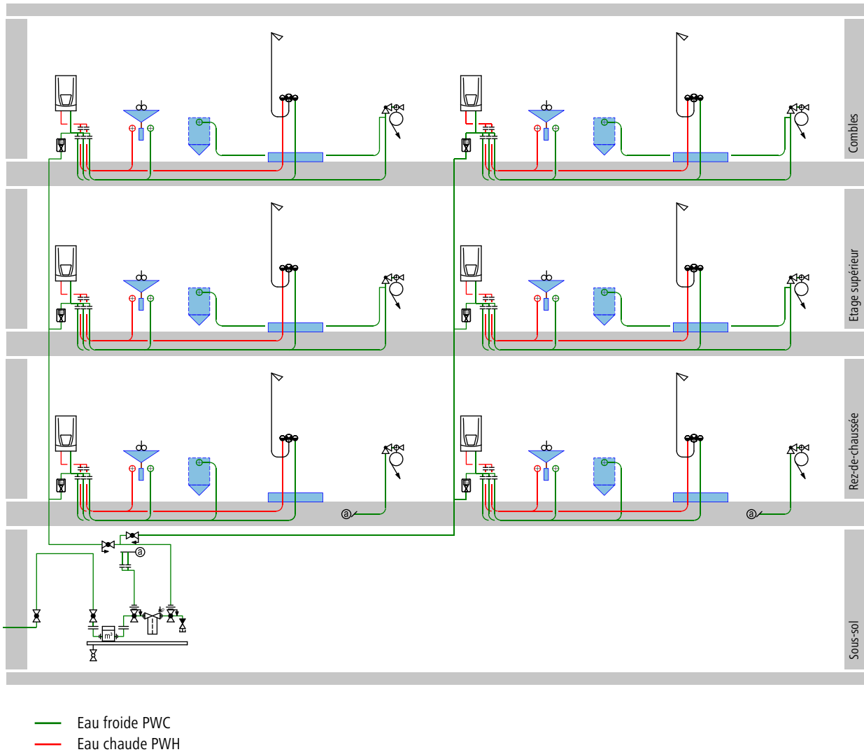
Fig. 22: Alimentation groupée avec chauffe-eau instantanés
