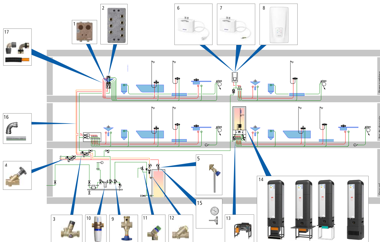
Fig. 45: Solutions Nussbaum pour l’approvisionnement en eau chaude
