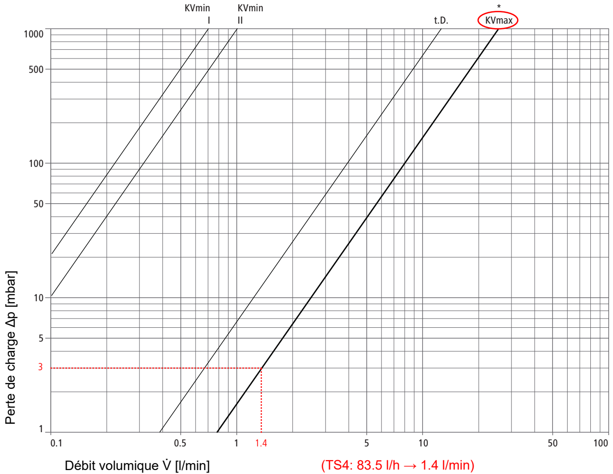
Fig. 47: Régulateur de circulation 36010: exemple de lecture du diagramme de performance
