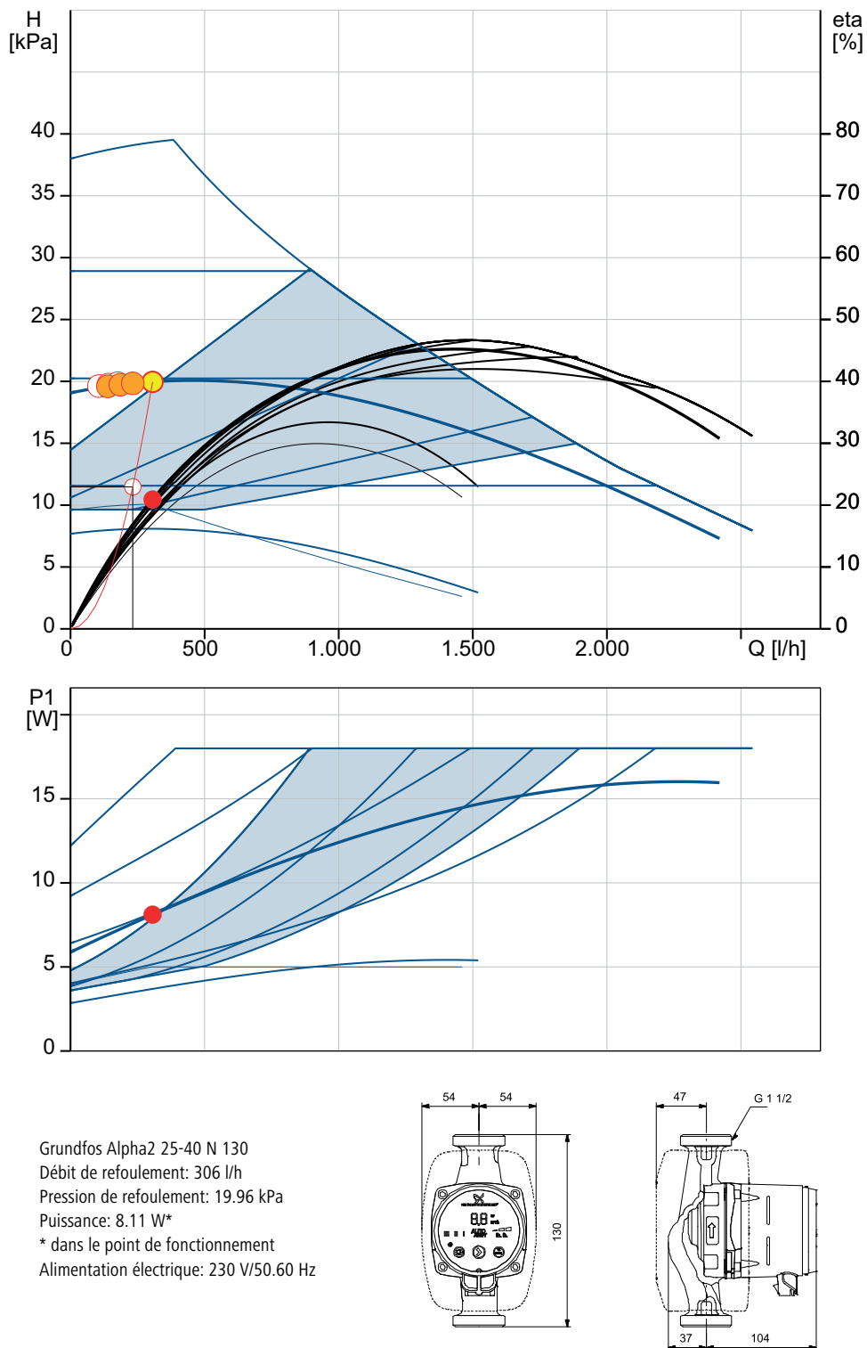
Fig. 48: Choix de la pompe de circulation à l'aide de l'outil de calcul du fabricant (figures: Grundfos)
