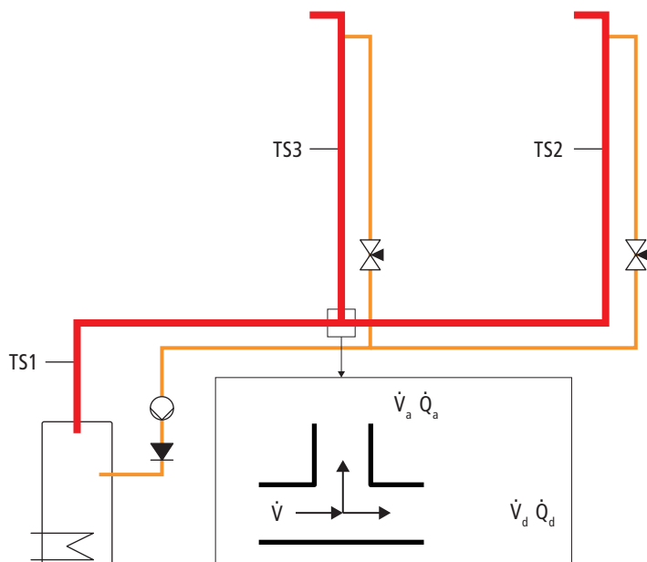
Fig. 38: Calcul des débits volumiques (selon le cours sur l'eau de Suissetec)
