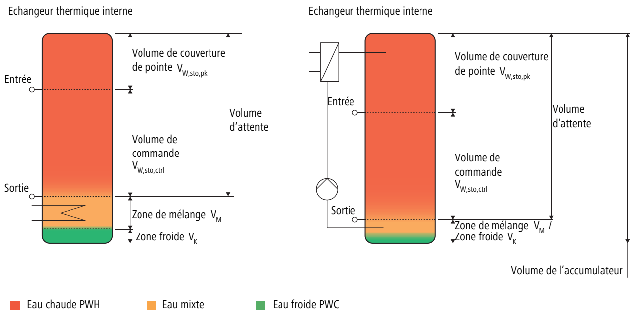
Fig. 15: Stratification dans le chauffe-eau à accumulation avec échangeur thermique interne et externe
