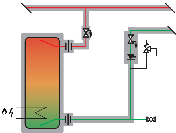
Fig. 10: Chauffe-eau à accumulation et chauffage direct
