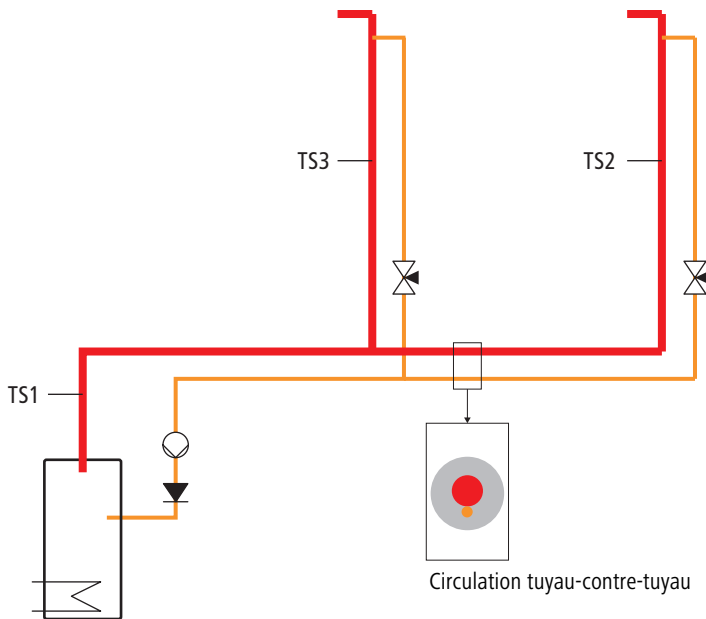
Fig. 37: Calcul de la circulation tuyau-contre-tuyau (selon le cours sur l'eau de Suissetec)
