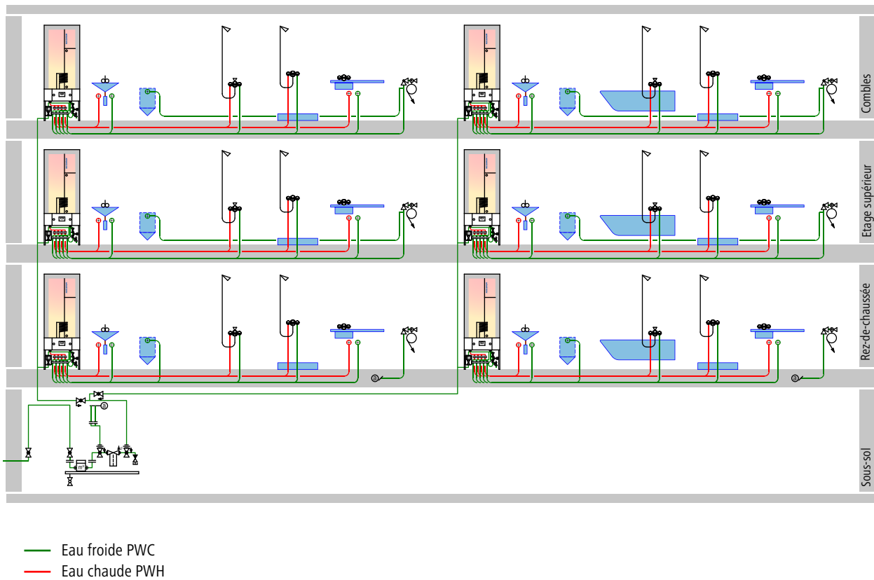
Fig. 23: Alimentation groupée avec chauffe-eau à accumulation
