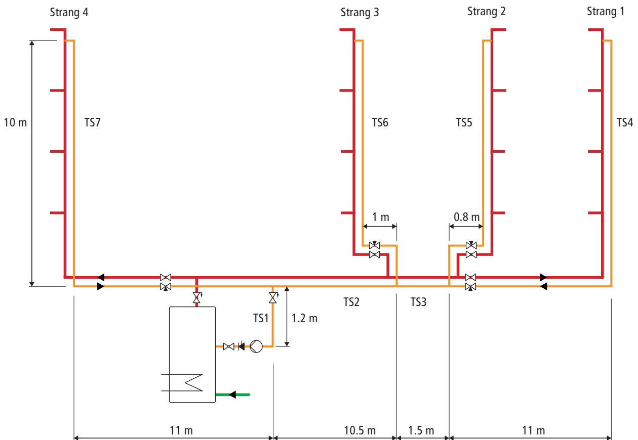
Fig. 40: Exemple de dimensionnement de la circulation d'eau chaude (selon le cours sur l'eau de Suissetec)
