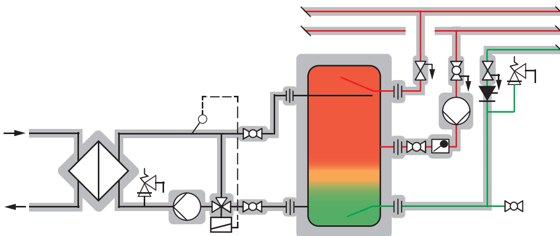
Fig. 12: Chauffe-eau à accumulation, chauffé indirectement avec un échangeur thermique externe
