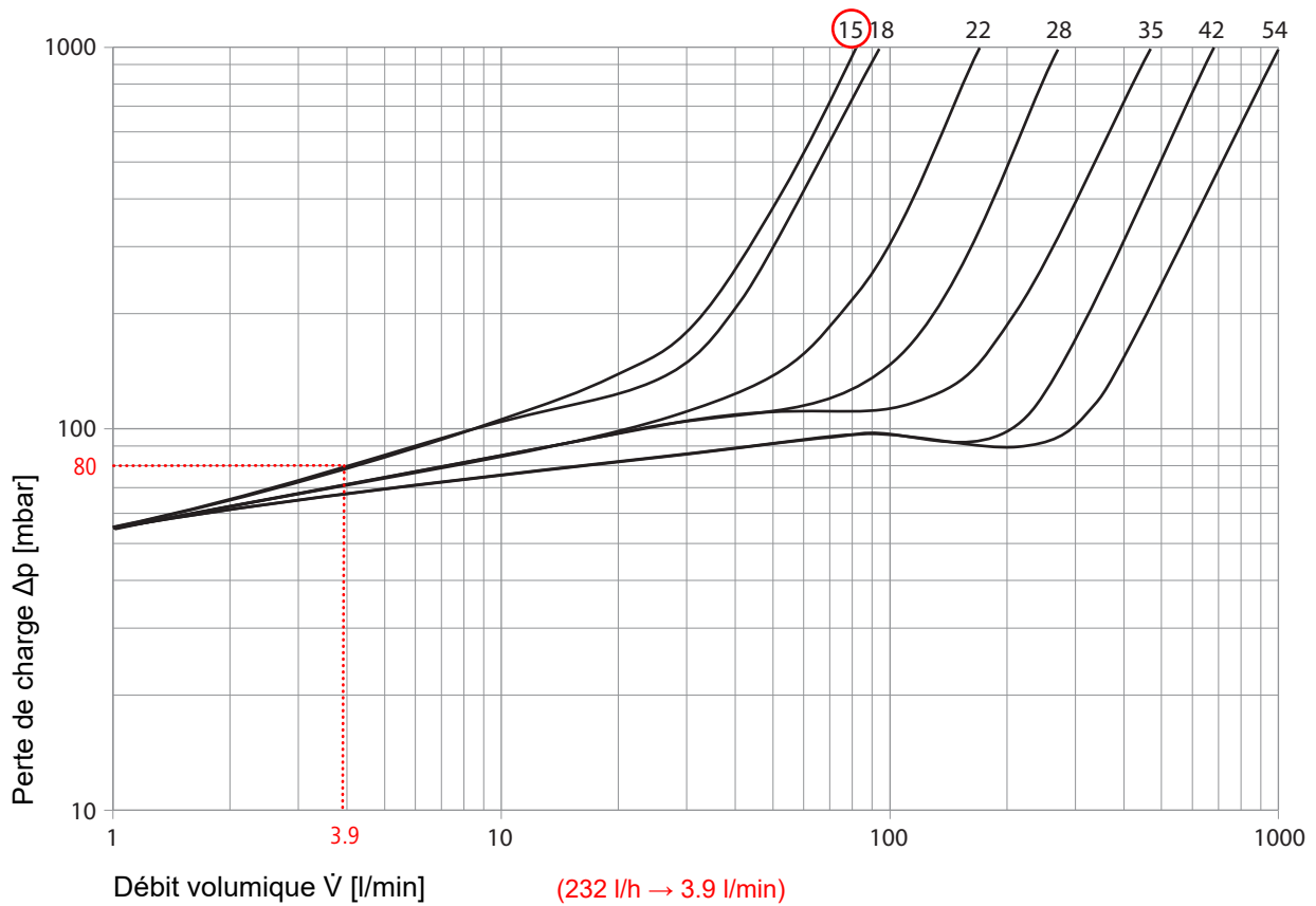
Fig. 46: Clapet anti-retour Optipress-Aquaplus 80189/81163: exemple de lecture du diagramme de performance
