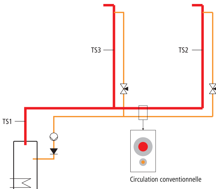
Fig. 36: Calcul de la circulation conventionnelle (selon le cours sur l'eau de Suissetec)
