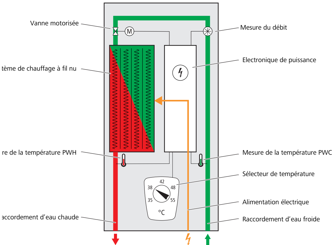
Fig. 18: Principe de fonctionnement d'un chauffe-eau instantané à régulation électronique
