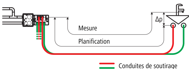
Fig. 43: Les valeurs calculées et mesurées des temps de soutirage peuvent différer en raison des pertes de pression \Delta p non prises en compte.
