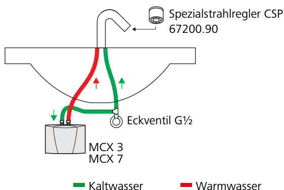
Abb. 21: Einzelversorgung mit den Waschtisch-Durchlauferhitzern MCX 3 / MCX 7
