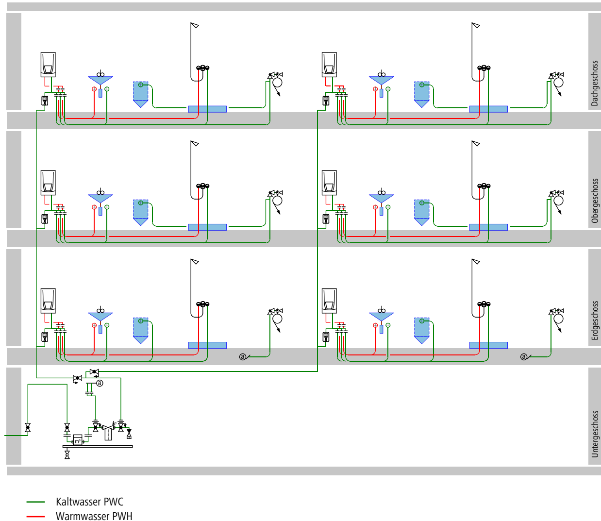
Abb. 22: Gruppenversorgung mit Durchlauf-Wassererwärmern
