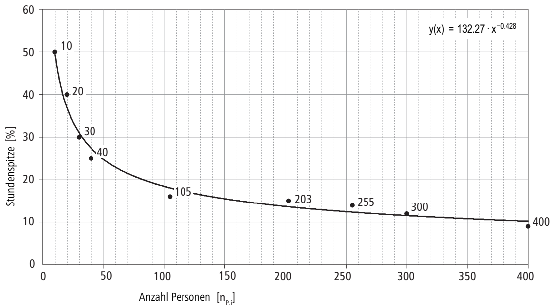
Abb. 35: Stundenspitze bei Wohnbauten mit > 10 Personen (nach Sanitärechnungen – kurz & bündig)
