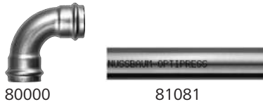
Abb. 4: Optipress-Aquaplus-Bogen 90° und Optipress-Edelstahlrohr 1.4520
