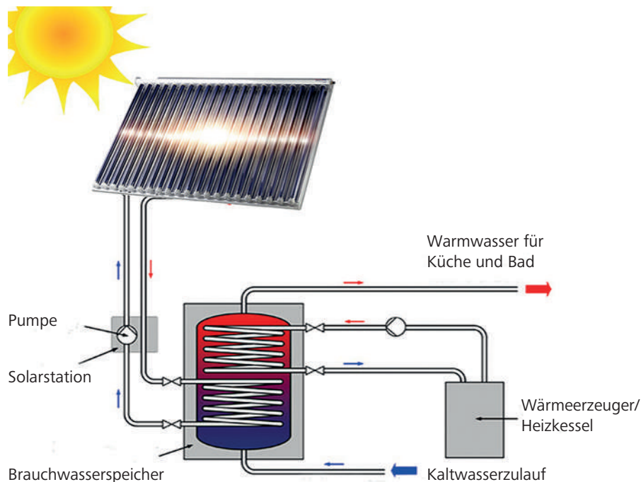
Abb. 1: Schematische Darstellung einer thermischen Solaranlage
