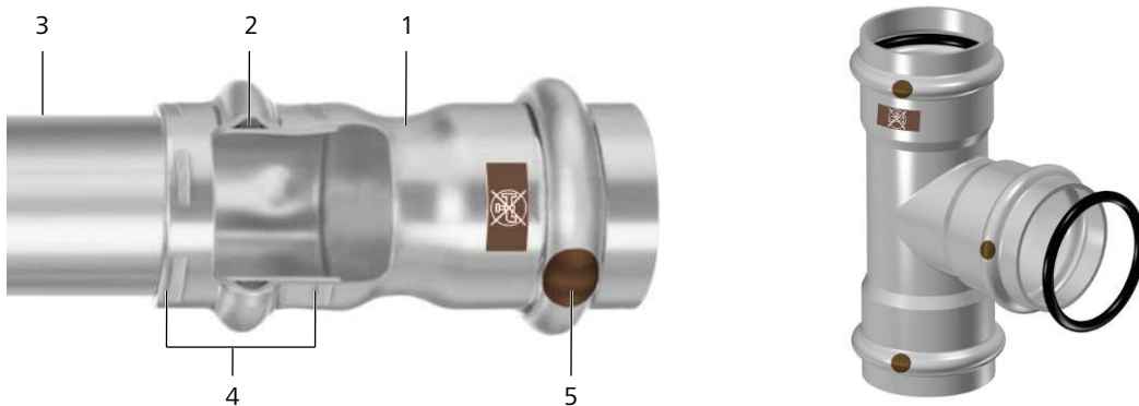
Abb. 2: Optipress-Industry-Pressverbindung Ø 15 bis 54 mm
