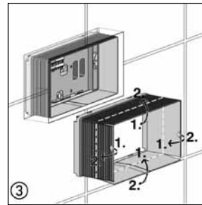
③ Seiten abknicken und entfernen. Der Rand des Revisionsschachtes muss mit der Wandoberfläche bündig sein. Rompre les côtés en les pliant et les éliminer. Le bord du cadre d'accès doit être à fleur du mur fini. Spezzare i lati piegandoli e rimuoverli. Il bordo del pozzo di revisione deve essere a raso con la superficie della parete.
