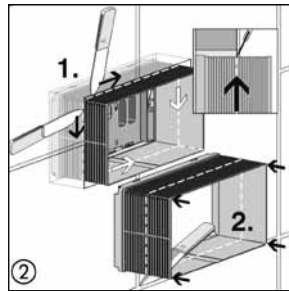
② Ecken des Revisionsschachtes bis zur Wandoberfläche einschneiden. Sectionner les angles du cadre d'accès jusqu'au mur fini. Intagliare gli angoli del pozzo di revisione fino alla superficie della parete.
