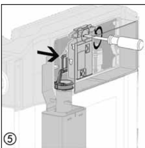
⑤ Arretierung der Mechanik lösen, Bügel des Ablaufventils aushängen. Libérer le mécanisme et le désaccoupler de l'étrier. Liberare l'arresto della meccanica - sganciare la stanghetta della valvola di scarico.
