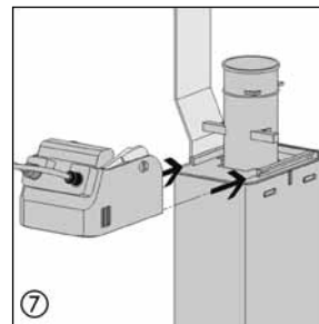
⑦ Bowdenzugseinheit von links auf das Ablaufventil schieben, bis es einrastet. Introduire le support de câbles Bowden depuis la gauche de la cloche jusqu'à enclenchement. Da sinistra spingere l'unità cavo Bowden sulla valvola di scarico fino all'arresto.
