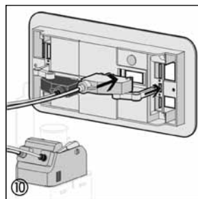
⑩ Die Kabelzüge in die Rückseite der Grundplatte einclippen. Grüner Bowdenzug auf die mit einem grünen Punkt markierten Stelle einclippen. Clipper les câbles Bowden au dos de la plaque de base (le câble de couleur verte à l'endroit marqué par un point vert).
