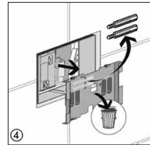
④ Abdeckung entfernen und Gewindebolzen herausnehmen. Die Abdeckung wird nicht mehr benötigt. Enlever le couvercle et retirer les tiges de fixation (éliminer le couvercle). Rimuovere la copertura e togliere i perni filettati. (La copertura non servirà più.)
