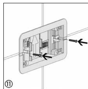
⑪ Grundplatte einsetzen und mit beiliegenden Schrauben befestigen. Mettre en place le cadre et le fixer avec les vis incorporées. Inserire la piastra base e fissarla con le viti allegate.
