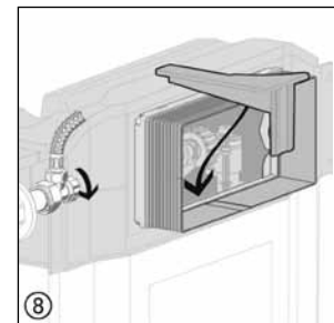
⑧ Halter wieder einsetzen und Eckventil öffnen. Remettre en place la cale de maintien et ouvrir le robinet équerre. Reinserrare il supporto e aprire la valvola ad angolo.
