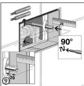
⑨ Die beiden Gewindebolzen in die Aufnahmebohrungen innerhalb des Revisionsschachtes einführen und durch 90°-Drehung fixieren. Dabei das angegebene Maß beachten: 20 mm Vorderkante Gewindebolzen-Vorderkante Wandoberfläche.
