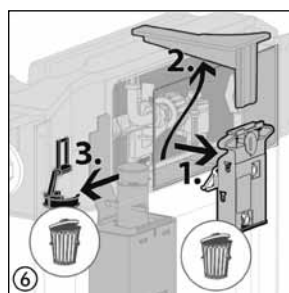
⑥ Mechanik entfernen, Halter herausnehmen. Bügel des Ablaufventils entfernen. Mechanik und Bügel werden nicht mehr benötigt. Extraire le mécanisme (1) et la cale de maintien (2). Retirer l'étrier (3) de la cloche (le mécanisme et l'étrier sont à éliminer). Rimuovere la meccanica, togliere il supporto. Rimuovere la stanghetta della valvola di scarico (la meccanica e la stanghetta non serviranno più).
