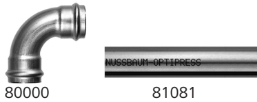
Fig. 4: Coude Optipress-Aquaplus 90° et tuyau en acier inoxydable Optipress 1.4520
