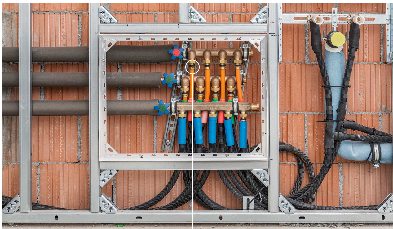
Fig. 7: Collegamenti Optiflex-Flowpress in una distribuzione sui piani montata
