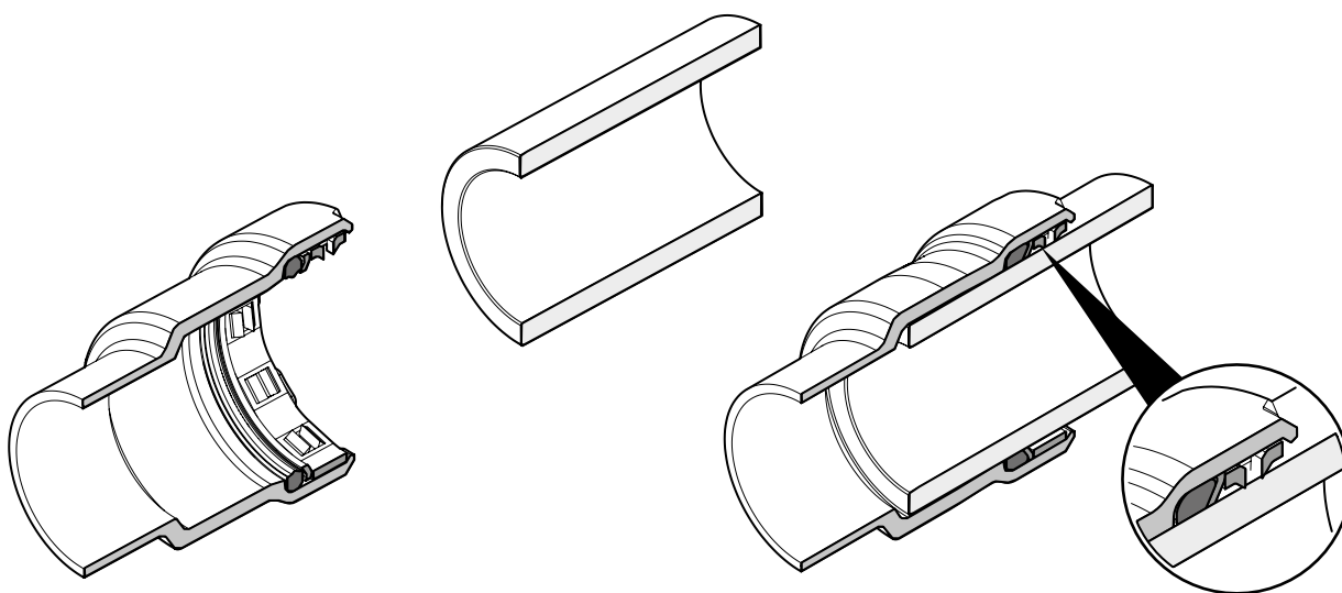
Fig. 5: Collegamento Optifitt-Press (aperto/pressato)
