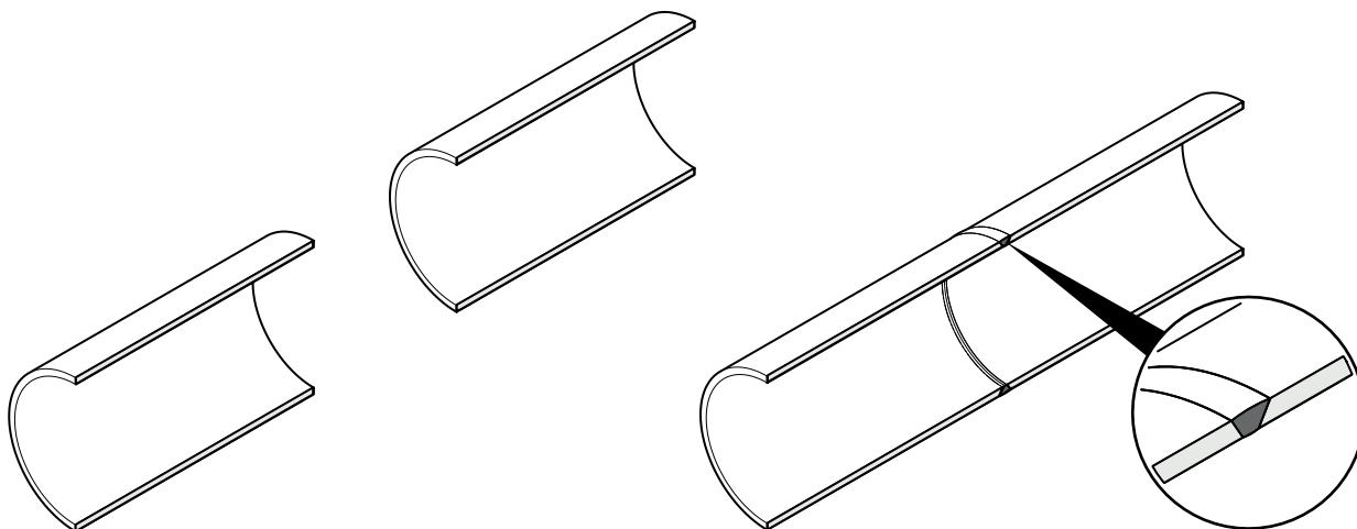
Fig. 18: Collegamento a saldare (aperto/saldato)
