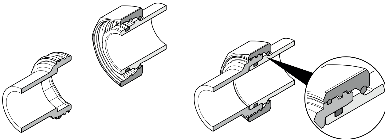
Fig. 10: Accoppiamento rapido (aperto/chiuso)
