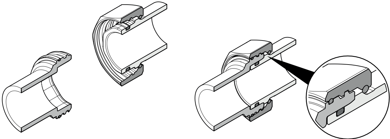
Fig. 10: Accouplement rapide (ouvert/fermé)
