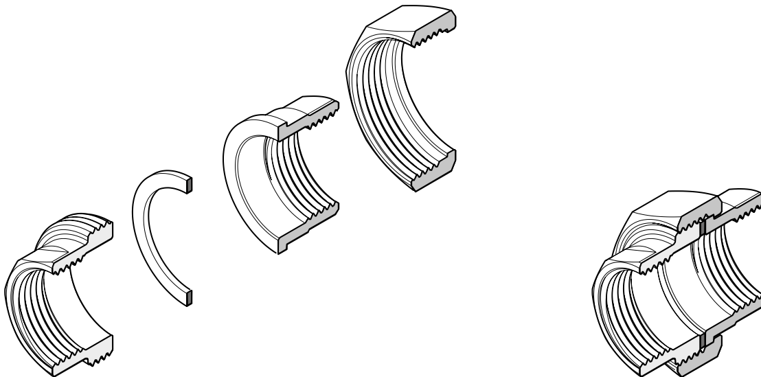
Fig. 13: Assemblage par filetage de tuyaux selon ISO 228-1 (non vissé/vissé)
