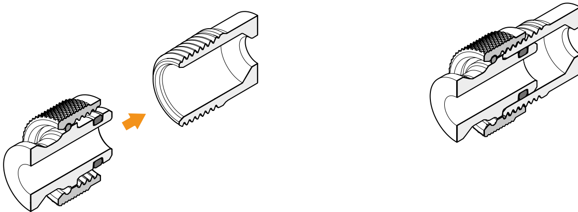
Fig. 17: Adaptateur MF (ouvert/fermé)
