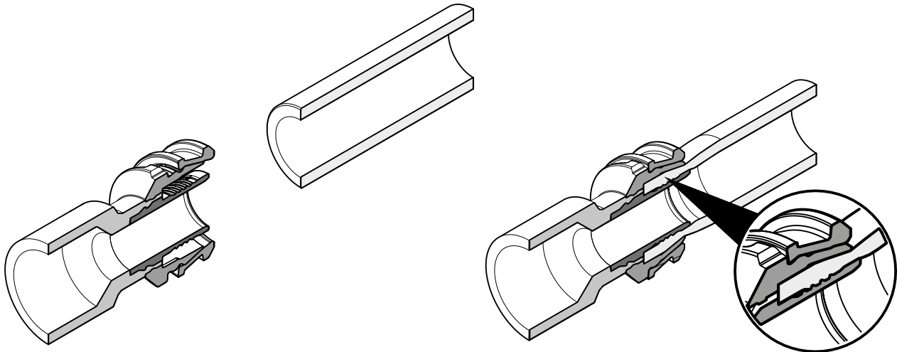
Fig. 6: Assemblage Optiflex-Flowpress (ouvert/serti)
