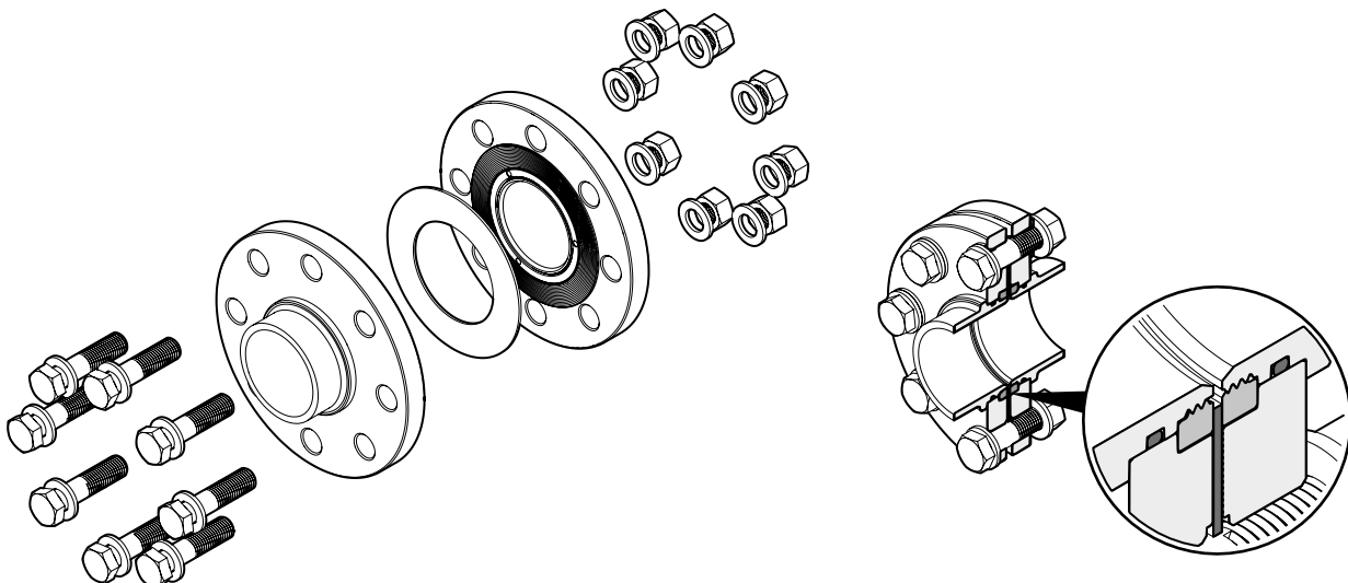
Fig. 15: Assemblage par bride tournante (non vissé/vissé)
