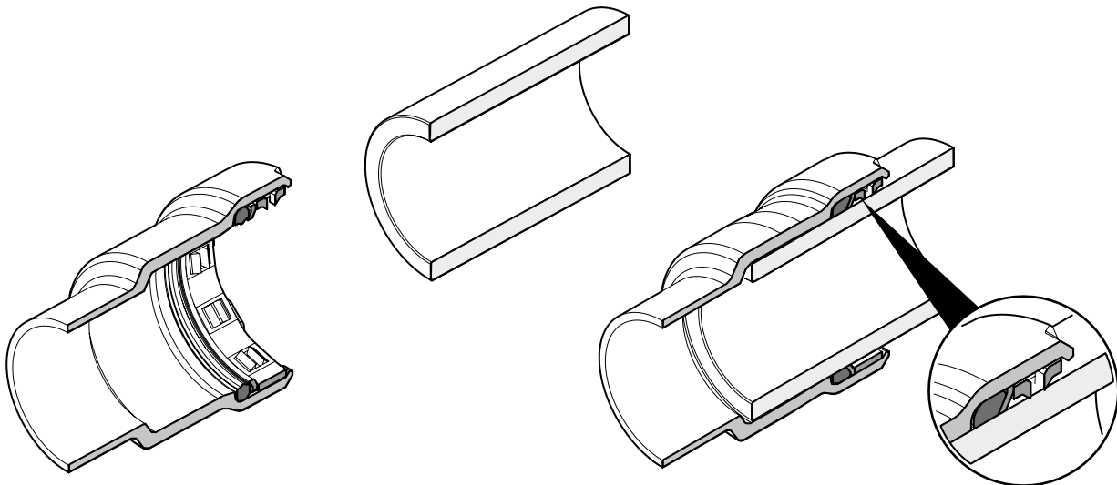
Fig. 5: Assemblage Optifitt-Press (ouvert/serti)
