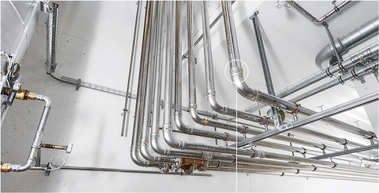
Fig. 4: Raccords à sertir montés avec assemblages Optipress-Aquaplus
