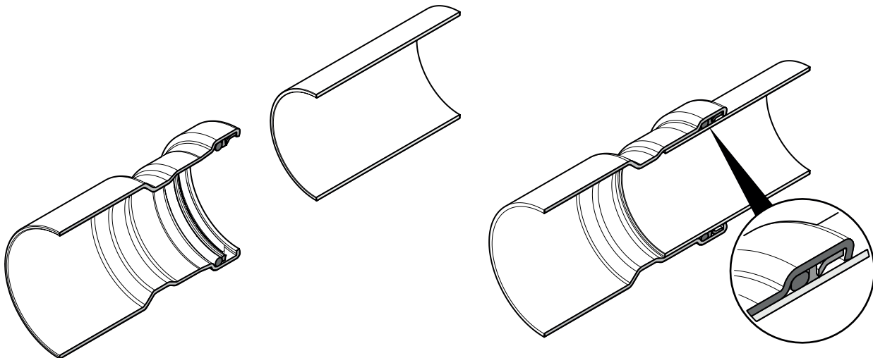
Fig. 3: Assemblage Optipress-XL (ouvert/serti)
