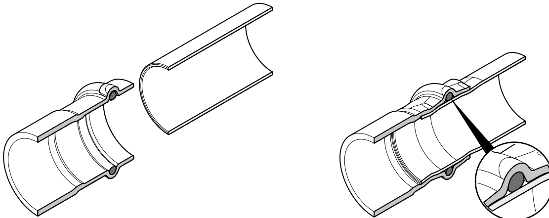
Fig. 1: Assemblage Optipress (ouvert/serti)
