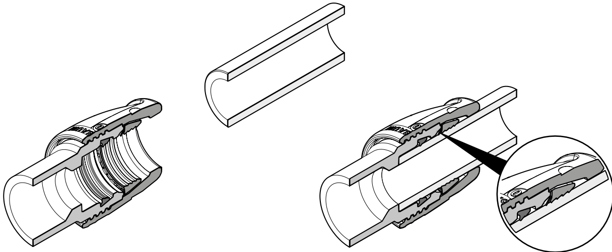
Fig. 8: Assemblage Optiflex-Profix (ouvert/emboîté)
