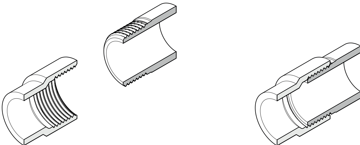
Fig. 12: Assemblage par filetage de tuyaux selon ISO 7-1/EN 10226 (non vissé/vissé)
