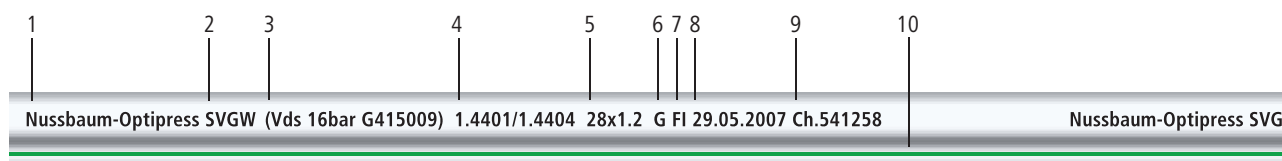
Fig. 1: Marquage du tuyau Optipress en acier inoxydable 1.4521
