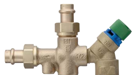
Mit Press-Verschraubungen für die Nussbaum-Systeme Optipress / Cupress.
