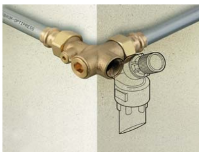
Die Stellung des Ecksicherheitsventils ist immer senkrecht.
