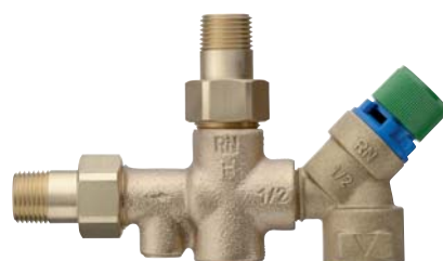
Mit Rohrverschraubungen für alle gängigen Systeme.
